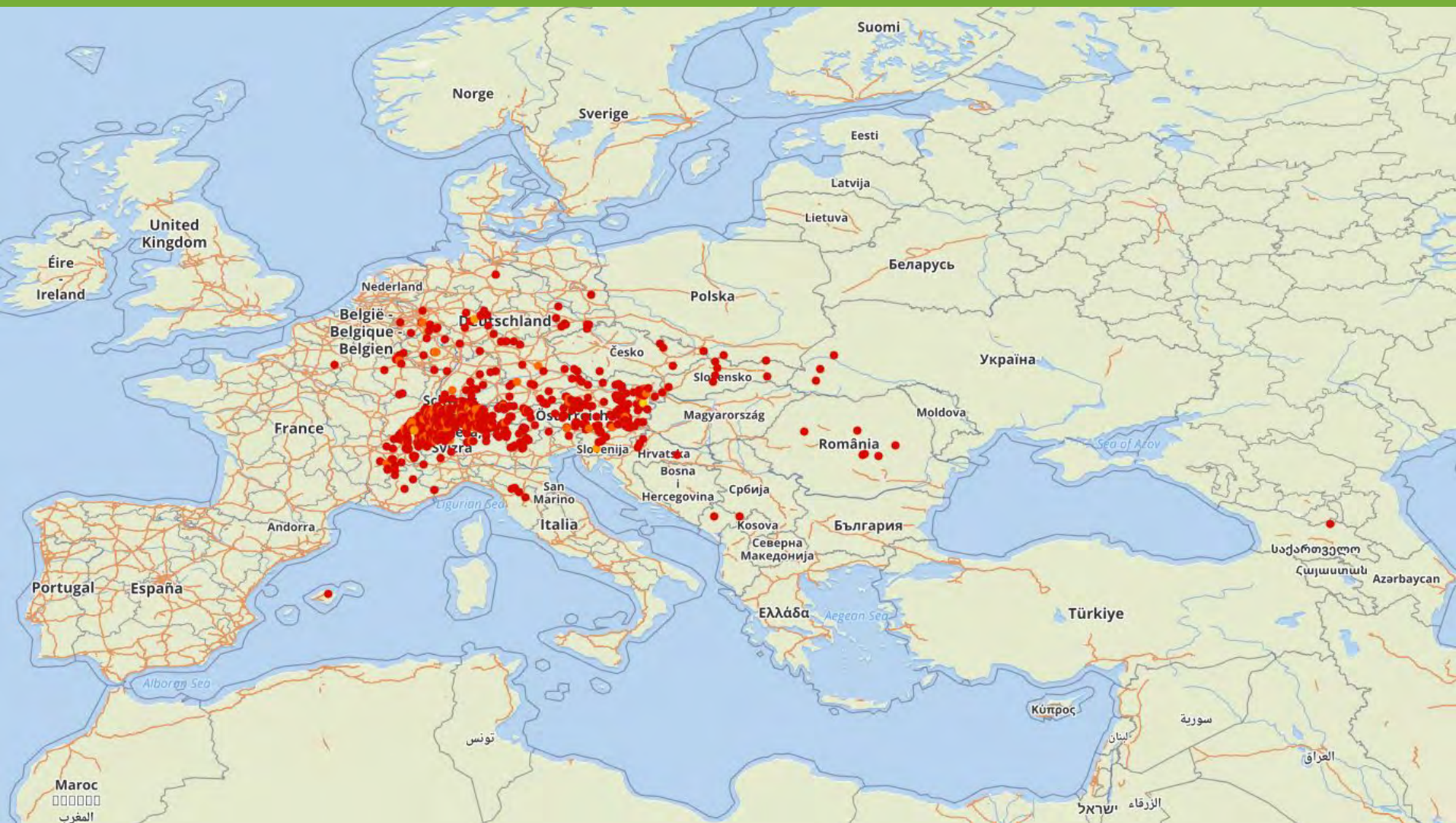
Répartition générale de Cicindela sylvicola Dejean, 1822
