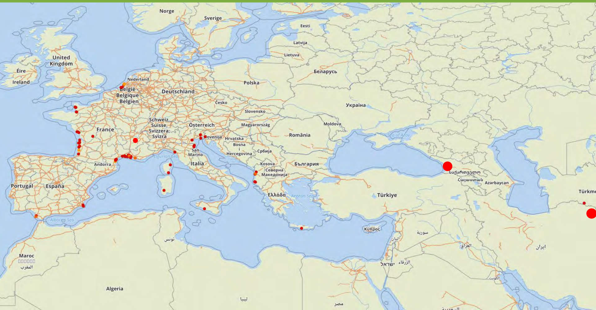
Répartition générale de Cylindera (Cylindera) germanica (Linné., 1758)
