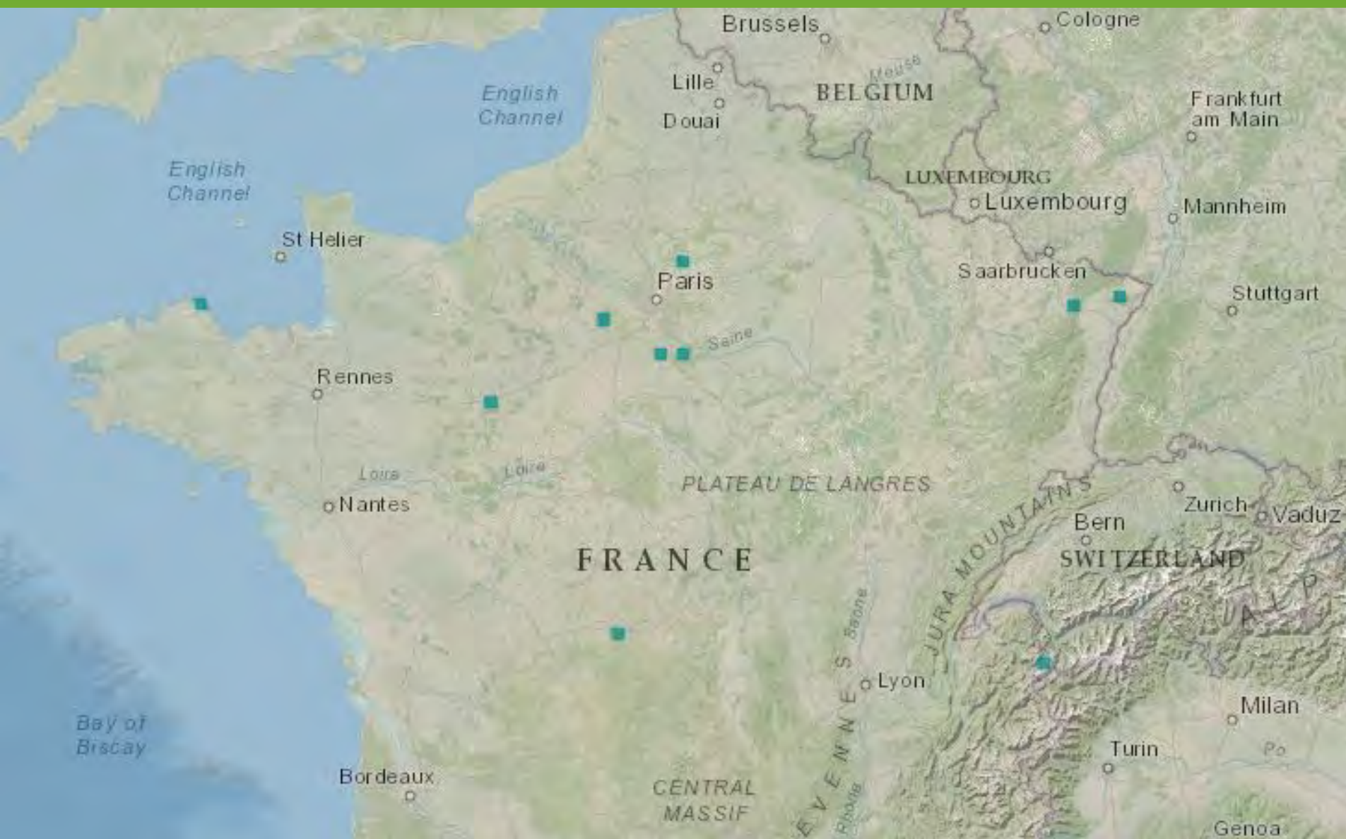
Répartition en France de Cicindela sylvatica Linnaeus, 1758
