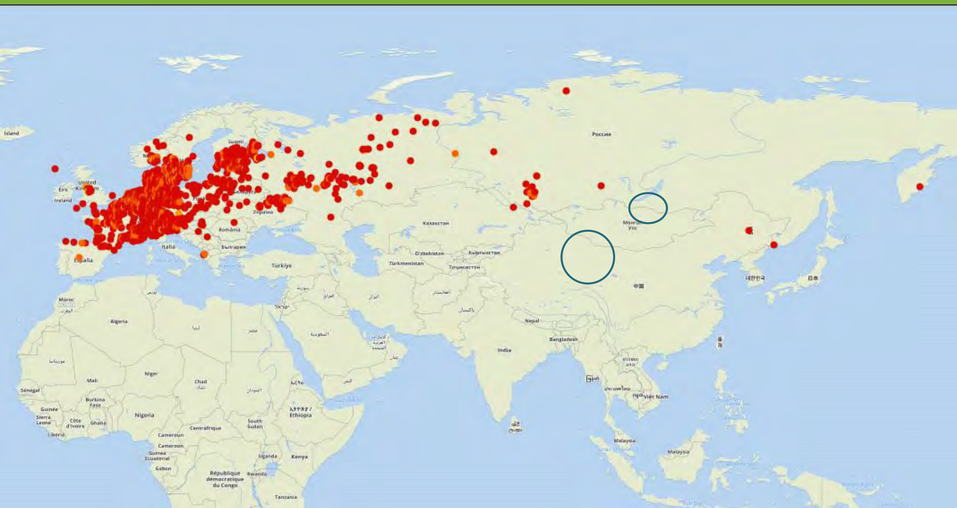
Répartition générale de Cicindela hybrida Linnaeus, 1758
