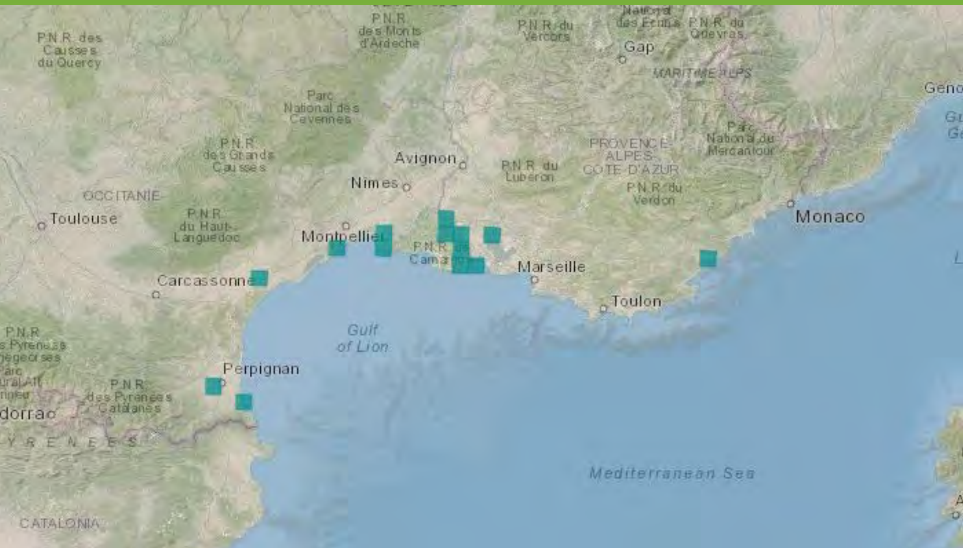
Répartition en France de Cylindera (Cylindera) paludosa (Dufour, 1820)
